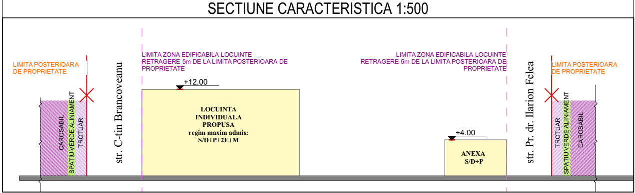
SECTIUNE CARACTERISTICA 1:500
